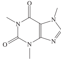
Caffeine
